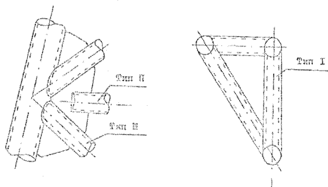
Рисунок 1. Типы соединений распорных и раскосных труб, рей и стоек мачты
