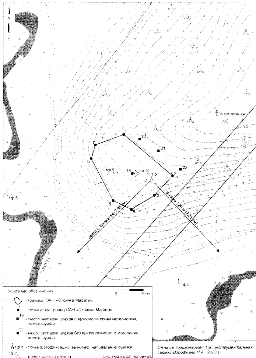
«Магистральный газопровод «Майя – Тунгюлю – Богоронцы Республики Саха (Якутия)» (III этап) (Республика Саха (Якутия)), Усть-Алданский район, Мегино-Кангаласский район. ОАН «Стоянка Марага». Инструментальный план.
