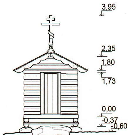
Западный фасад. М 1:100.
