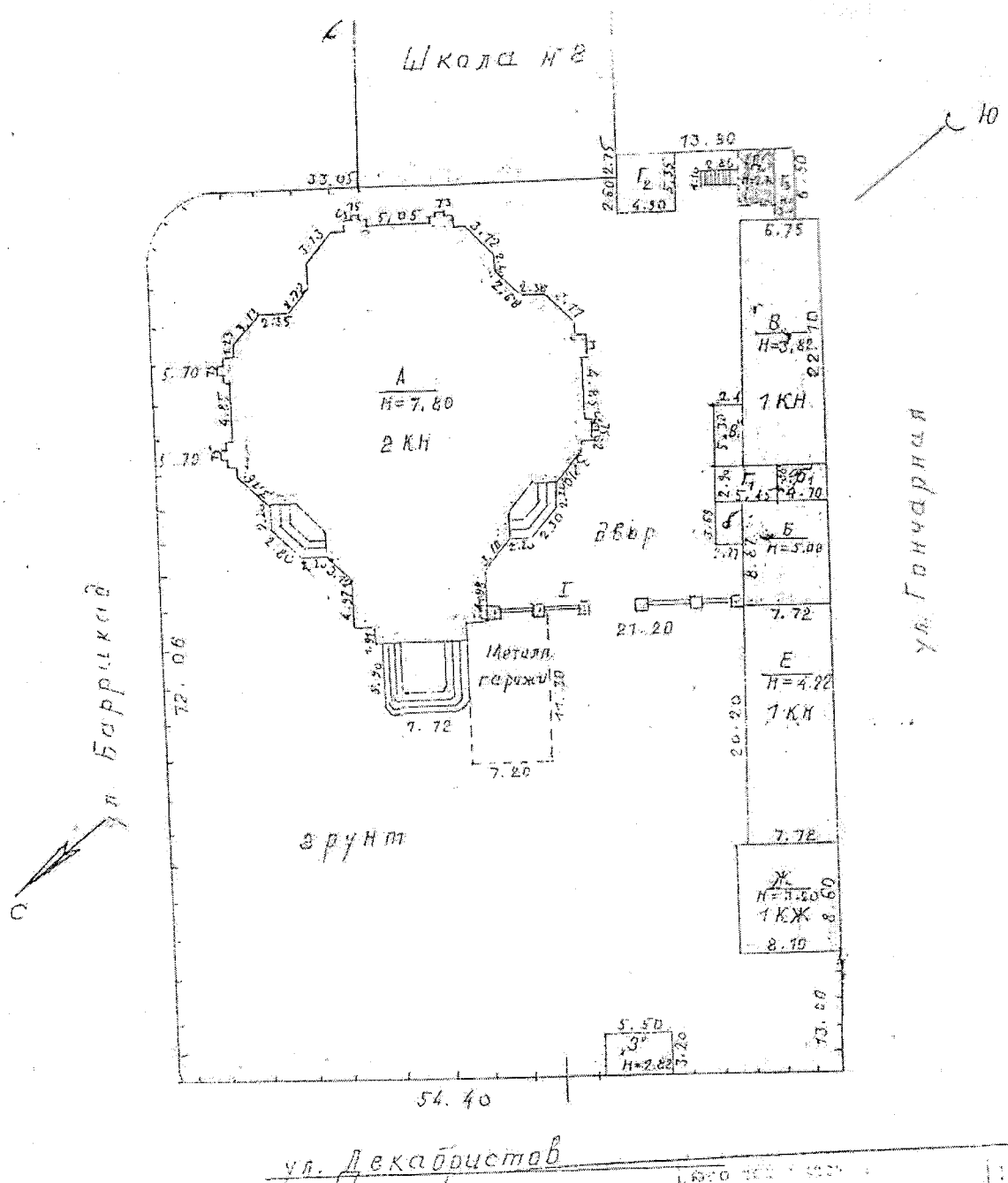
Рис. 1 - Схема генплана объекта
