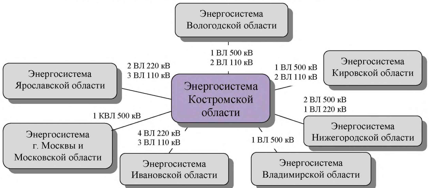
Схема внешних электрических связей Костромской области
