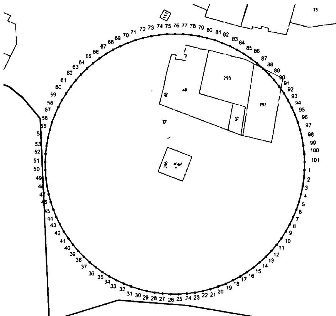
Координаты характерных точек границы третьего пояса ЗСО скважины в д. Яровская
