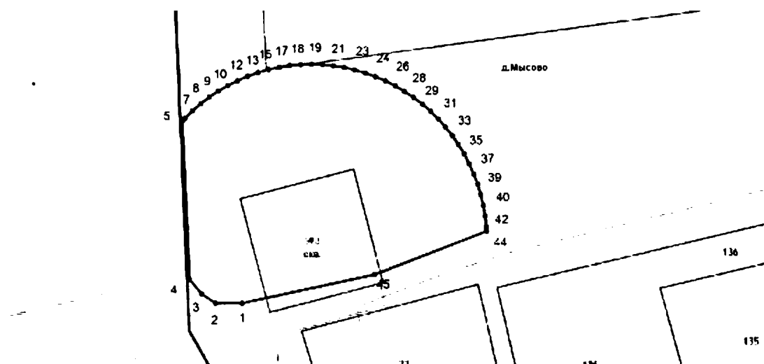
Координаты характерных точек границы первого пояса ЗСО скважины в д. Мысово
