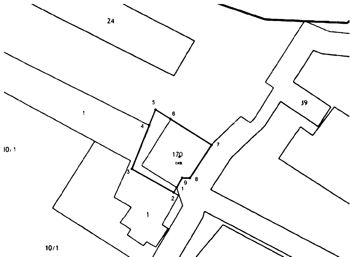
Координаты характерных точек границы первого пояса ЗСО скважины в д. Авдеево
