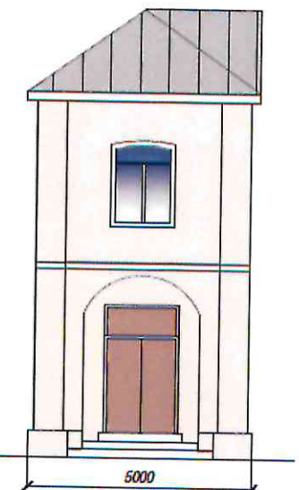
Вариант фрагмента фасада 3.2
