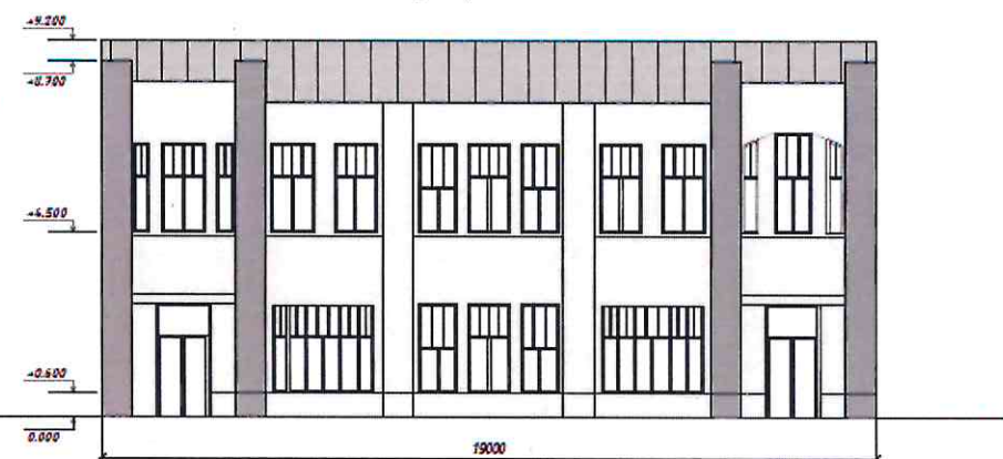
Вариант фасада 1.4
