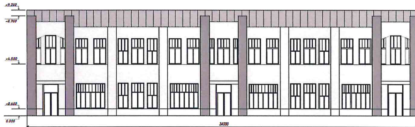
Вариант фасада 1.1
