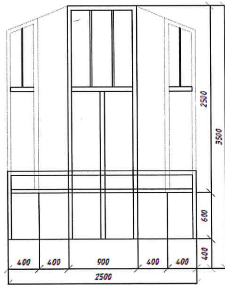
Вариант балкона
