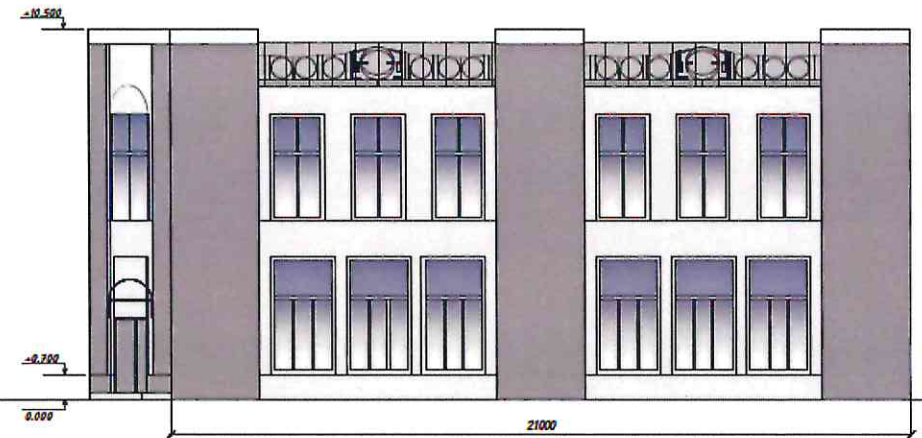
Вариант фасада 2.2
