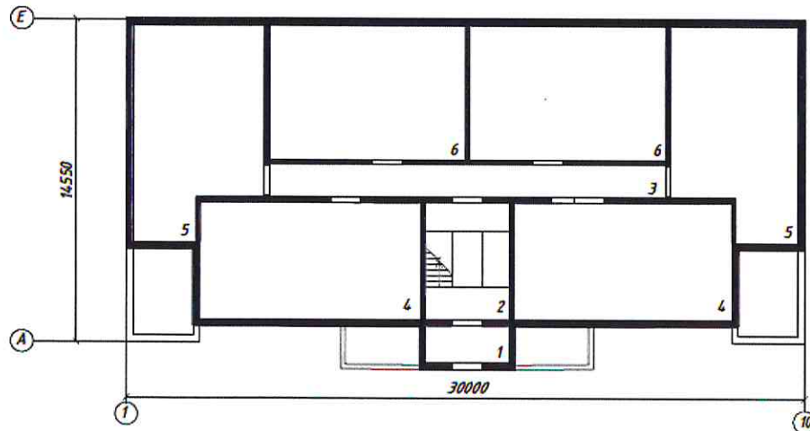
Планировочная схема 2-ого этажа здания коридорного типа М 1:200
