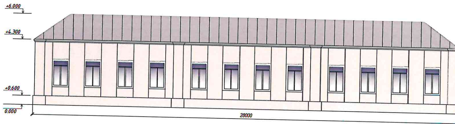
Вариант фасада 1, 2
