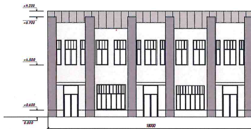
Вариант фасада 1.3
