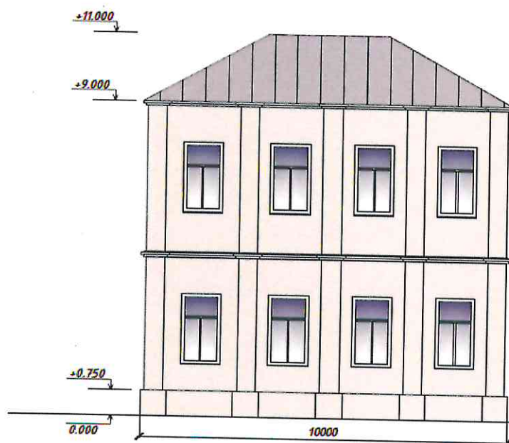
Вариант фасада 5
