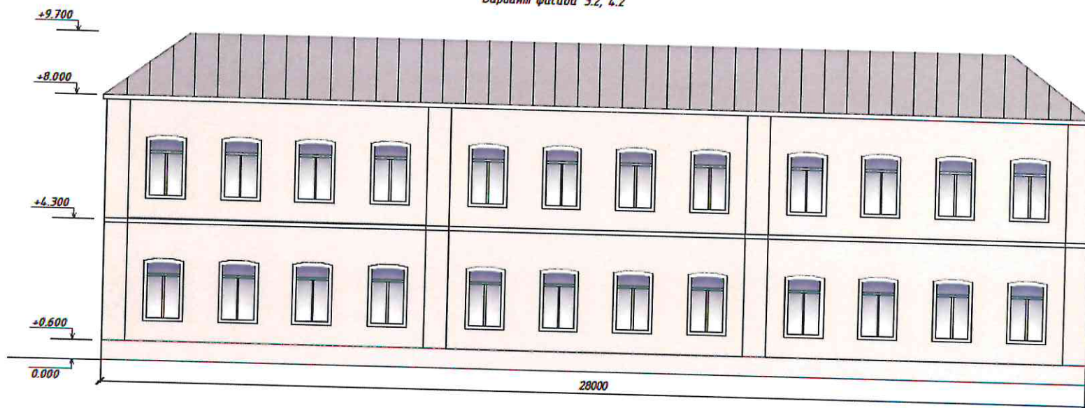
Вариант фасада 3.2, 4.2
