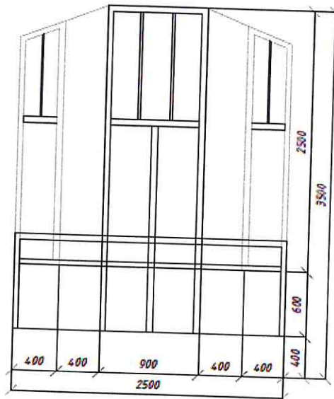
Вариант балкона
