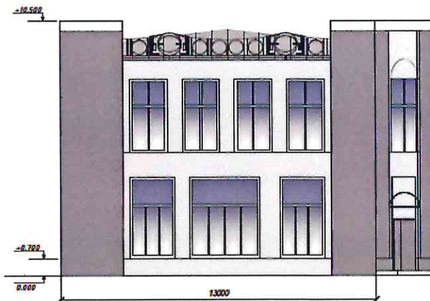
Вариант фасада 2.2
