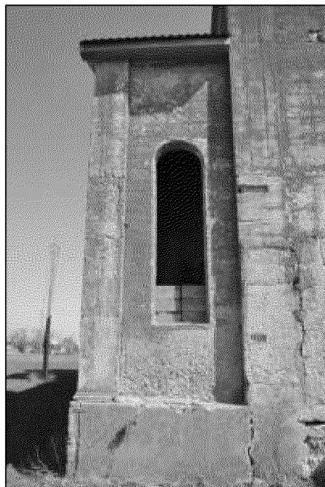
фрагмент западного фасада объекта культурного наследия (угловая лопатка, арочный оконный проем притвора, кордон цоколя)
