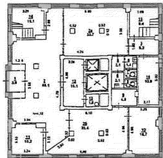
план третьего этажа
