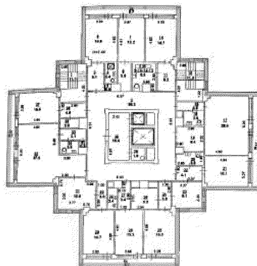
план шестого этажа
