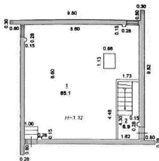
план мезонина
